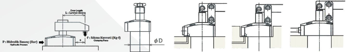
Montaj Şekilleri / Mounting Types
